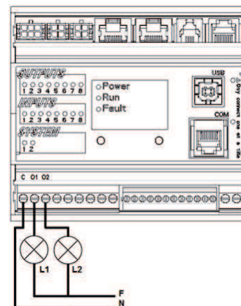
Рисунок 13: Пример соединений выходов со станцией I/O
