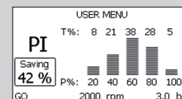
7.1.9 - Си Рисунок 18: Визуализация гистограммы мощности
