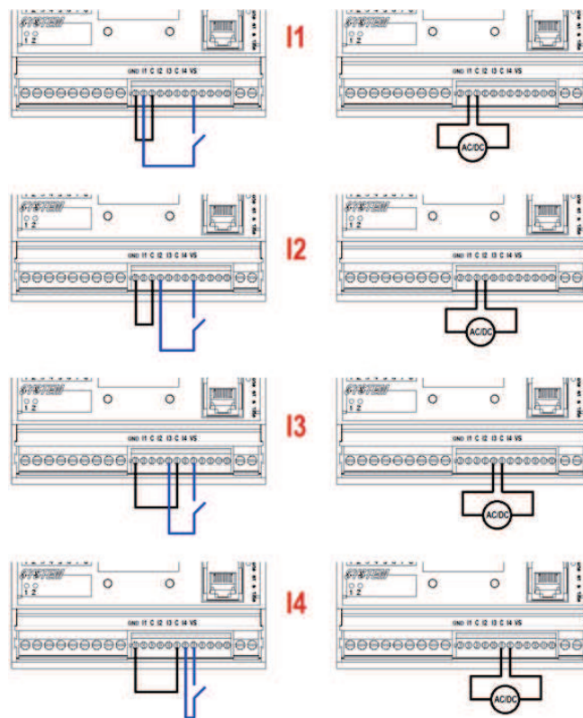
Рисунок 14: Пример соединения входов со станцией I/O
